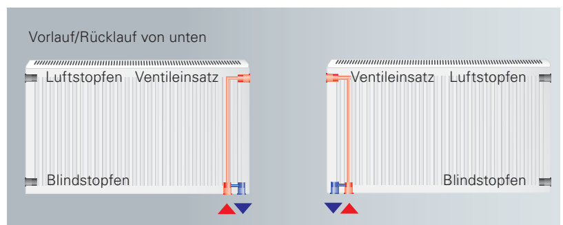
Ventilheizkörper Anschlussvarianten als Ventilheizkörper
