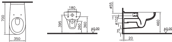
Wand-Tiefspül-WC spülrandlos mit Flush-Technologie, verlängert 700 mm
