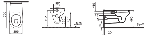
Flachspül-WC verlängert 700 mm
