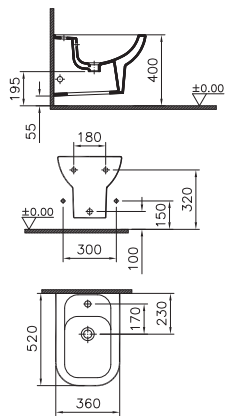
Bidet 52 cm, wandhängend, Wasseranschlüsse seitlich
