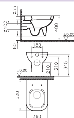
Tiefspül-WC 52 cm, wandhängend
