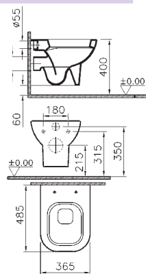
Tiefspül-WC Compact 48 cm, wandhängend
