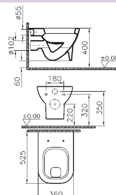
Flachspül-WC 52 cm, wandhängend
