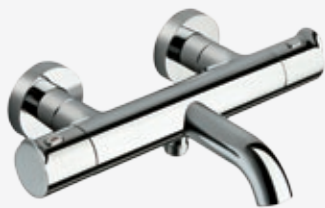
Wannen-Thermostat Aufputz Armaturenkörper mit Verbrühungsschutz, Breite 29 cm, Ausladung 18,5 cm (Wand bis Mitte Perlator)
