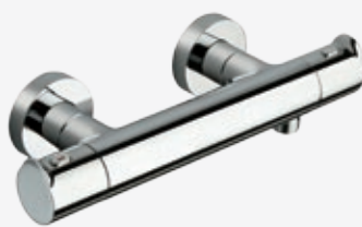
Brause-Thermostat Aufputz Armaturenkörper mit Verbrühungsschutz, Breite 29 cm, Ausladung 8 cm (Wand bis Mitte Auslauf)
