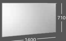
LICHTSPIEGELELEMENT* B 1400 / H 710 / T 55 mit Sensorschalter (dimmbar) und Anti-Beschlag (53 W) Direkte Beleuchtung: 52 W, 3575 lm Indirekte Beleuchtung: 46,6 W, 2660 lm Lichtspiegelement 807340000
