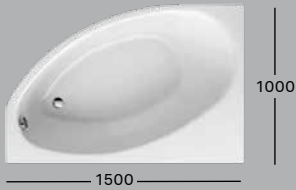
ASYMMETRISCHE ECKWANNE, RECHTS T 440 L 1500 / B 1000
