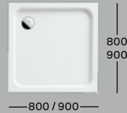
QUADRATISCHE DUSCHWANNE T 60 L 800 / B 800 L 900 / B 900
